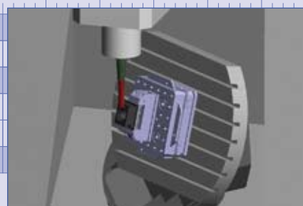
CAM-Programmierung und Simulation CAM programming and simulation
